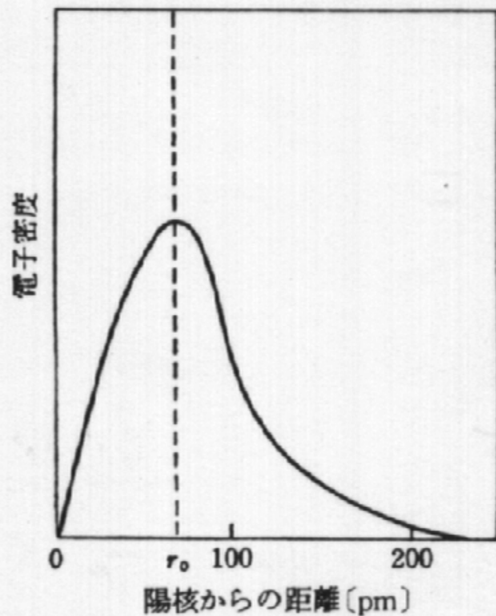
図 1・3 水素における電子の存在確率
