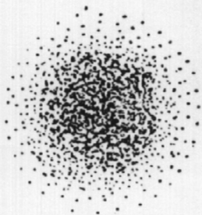
図 1・2 水素原子
